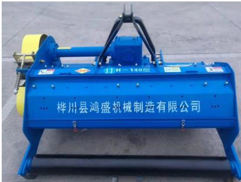
1JH-140 型秸秆粉碎还田机
